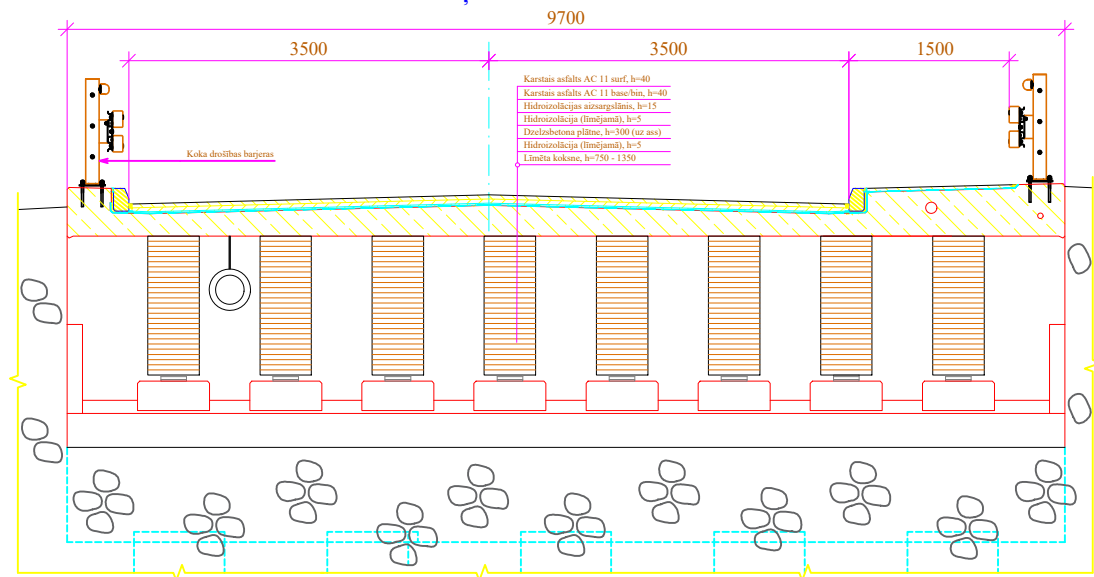
TILTA ŠĶĒRSGRIEZUMS
